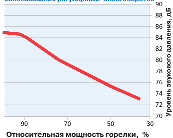
Уровень акустического шума в случае использования регулировки числа оборотов
